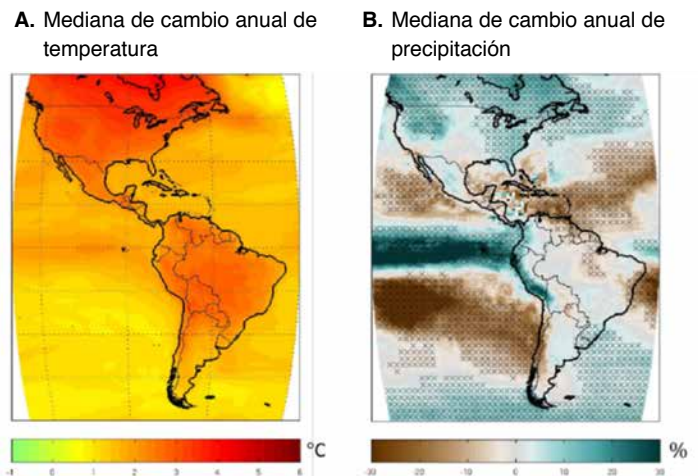
Fig. 1 – Mediana de cambios proyectados en 21 modelos climáticos NEX-GDDP a escala reducida para el escenario RCP8.5 (altas emisiones) a mitad del siglo (2040-2069) en comparación con la línea base de 1980-2005 para (a) temperatura anual; y (b) precipitación anual. Las marcas en (b) indican áreas en donde al menos el 70% de los modelos concuerdan en la dirección del cambio en precipitación (todas las regiones concuerdan fuertemente en cuanto al calentamiento en (a)). El calentamiento es más fuerte en tierra, aunque hay diferencias regionales en la tasa de calentamiento y los cambios en la precipitación. Obsérvese que los modelos individuales muestran una amplia gama de resultados potenciales húmedos y secos para muchas regiones.
